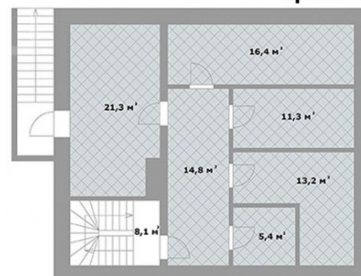
Цоколь
