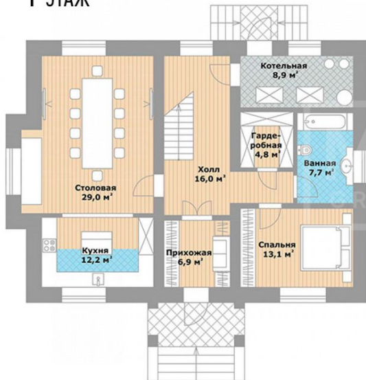
1 ЭТАЖ
