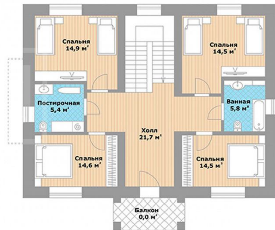
2 ЭТАЖ
