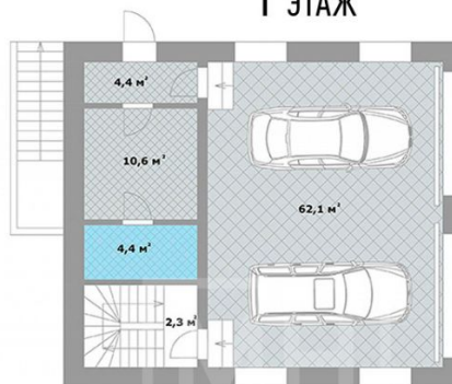
1 ЭТАЖ
